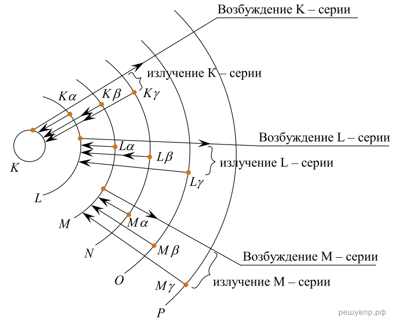
Рис. 2а. Схема образования линий характеристического спектра
