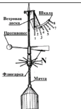
Рис. 2. Флюгер-анемометр Вильда
